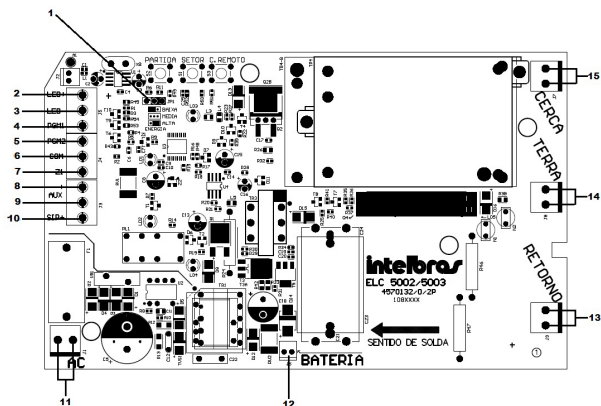
Visão interna da placa
